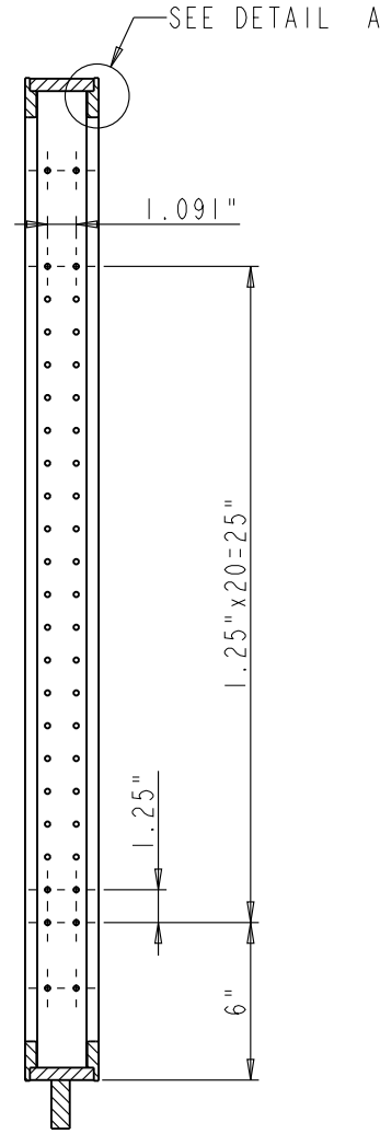
SECTION A-A
